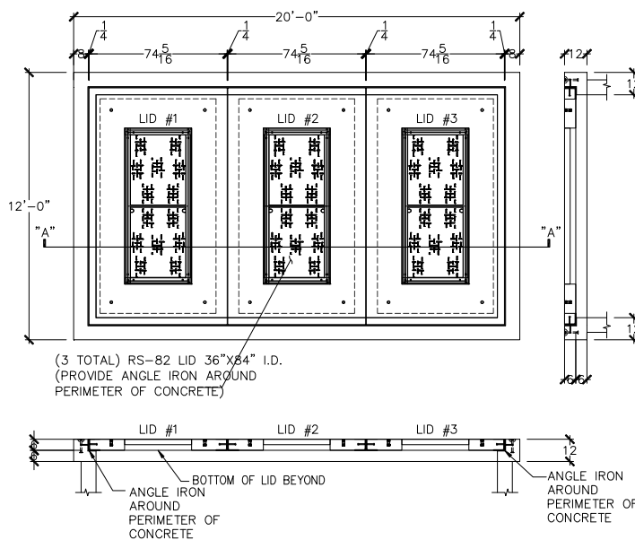
RS-82 LID PLAN
